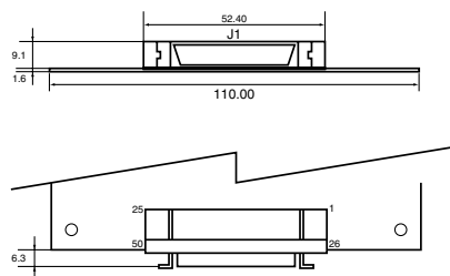
ACB-MDR50/MR寸法
