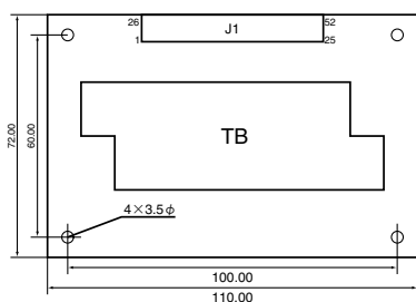
ACB-MDR50/MS寸法
